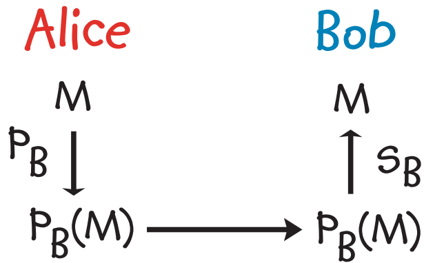
図 2.1: Briskorn の公開鍵 P_B によって暗号化された文は, Briskorn の秘密鍵 S_B でしか復号化できない
