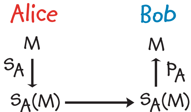
図 2.2: Abel の秘密鍵 S_A によって暗号化された文は, Abel の公開鍵 P_A でしか復号化できない
