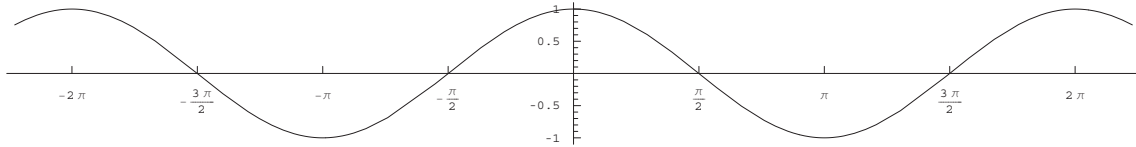
図 4.2: y = \cos x のグラフ
