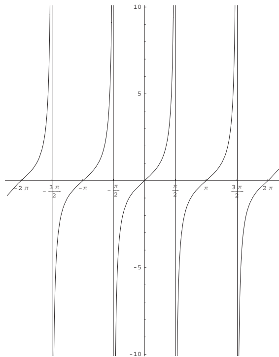
図 4.3: y = \tan x のグラフ
