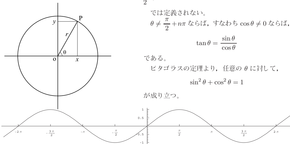
図 4.1: y = \sin x のグラフ
