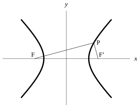
図 4: 双曲線の幾何学的定義
