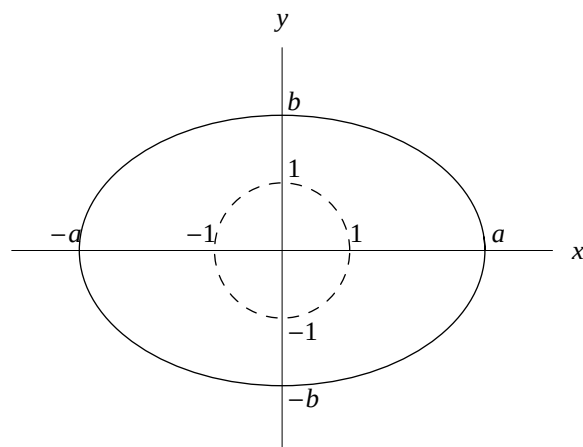
図 2: 円の 1 次変換
