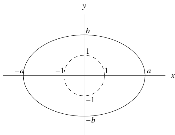
図 2: 円の 1 次変換
